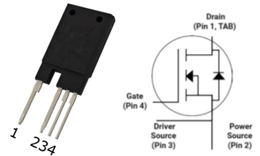
TO-247 Plus -4L
