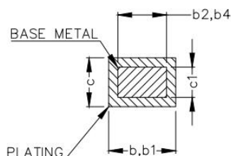
SECTION "F-F", "G-G" SCALE: NONE
