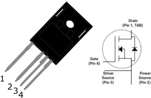
TO-247-4L
