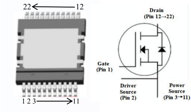
QDPAK-22L
