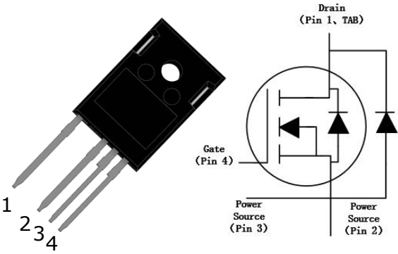
TO-247-4L
