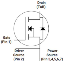
TO-263-7L
