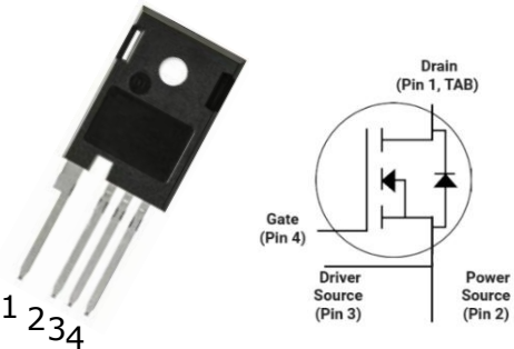
TO-247-4L
