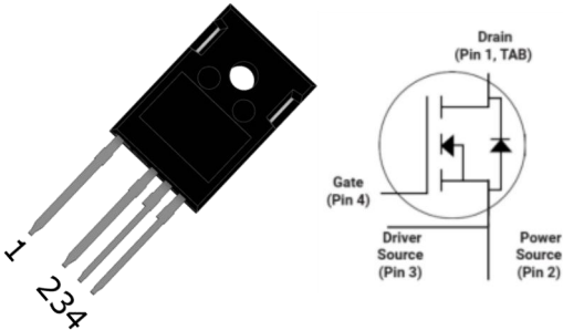
TO-247-4L
