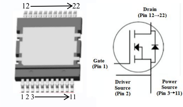
QDPAK-22L
