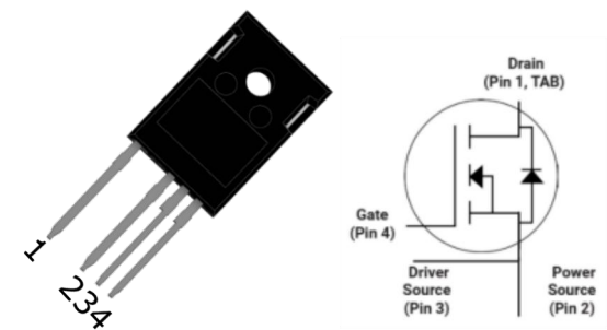
TO-247-4L
