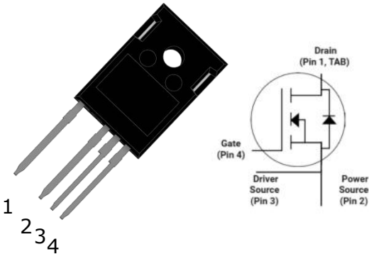
TO-247-4L
