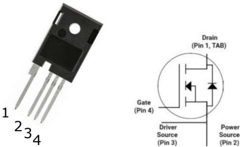
TO-247-4L
