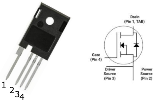
TO-247-4L
