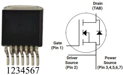
TO-263-7L
