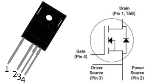
TO-247-4L
