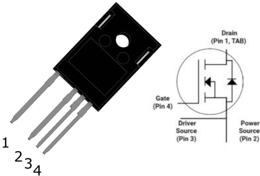
TO-247-4L
