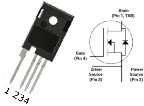
TO-247-4L
