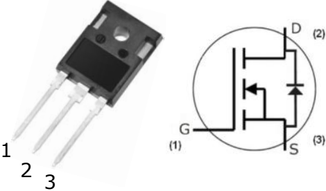
TO-247-3L
