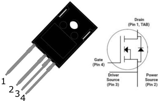
TO-247-4L
