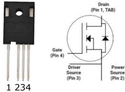
TO-247-4L
