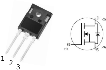
TO-247-3L
