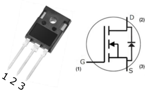
TO-247-3L
