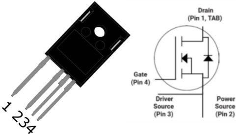
TO-247-4L
