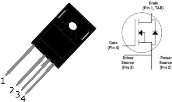
TO-247-4L
