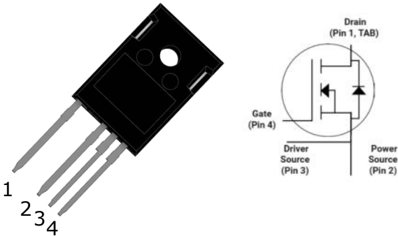
TO-247-4L
