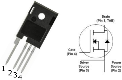
TO-247-4L
