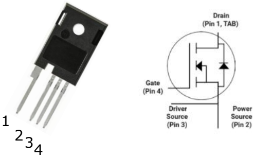
TO-247-4L
