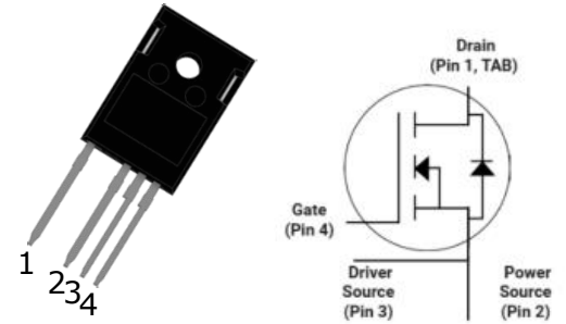
TO-247-4L
