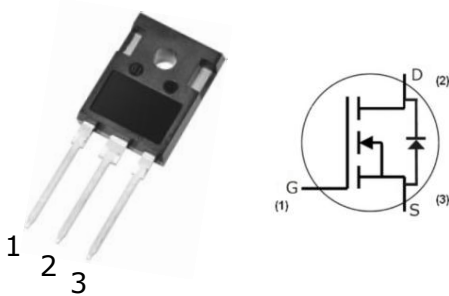
TO-247-3L
