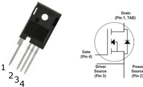
TO-247-4L
